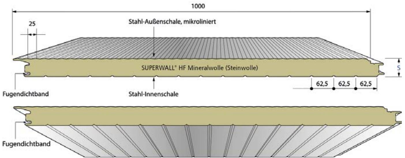
Deckschalenvarianten auf Anfrage, Maße in mm
